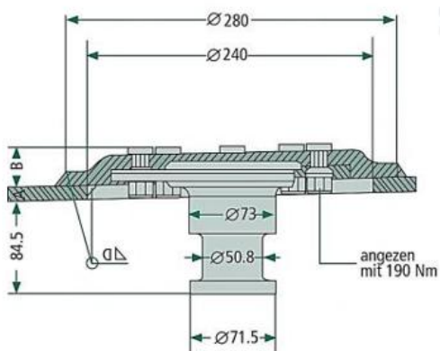
Fig. 04. Modelo de King pin y sus dimensiones en milímetros y pulgadas.
